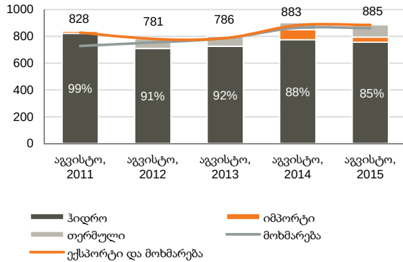
გრაფიკი 1: ელექტროენერგიის წარმოება და მოხმარება, გვტ/სთ
