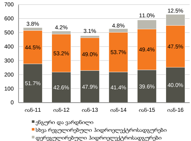
გრაფიკი 4: ჰეს-ების გამომუშავება, გვტ/სთ
